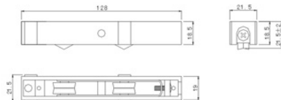
型号：PWS24# 尼龙座调节双轮
